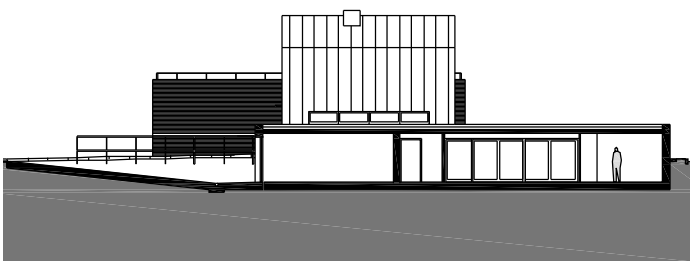
langsdoorsnede
